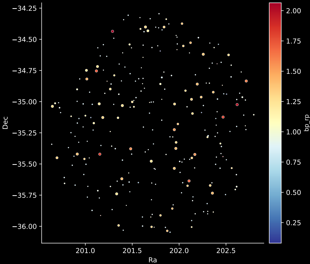
GALAH DR4 Field: [2848] Stars: 263
