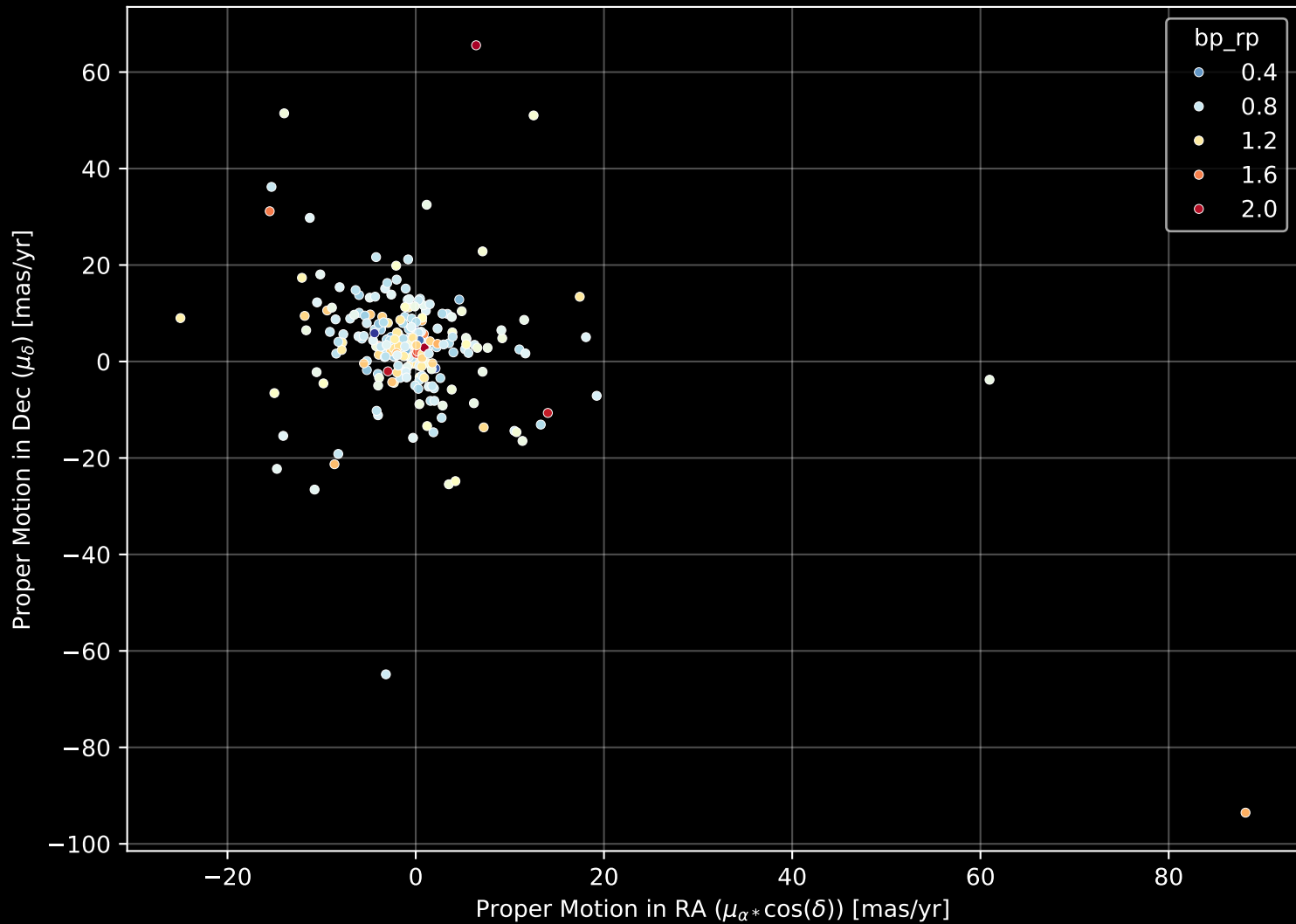
GALAH DR4 Field: [2848] Proper Motion Diagram (n= 263)
