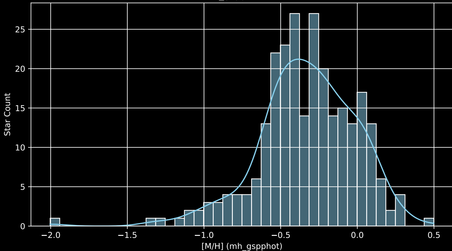
GALAH DR4 Field: [2848] [M/H] (mh_gspphot) (n= 263)
