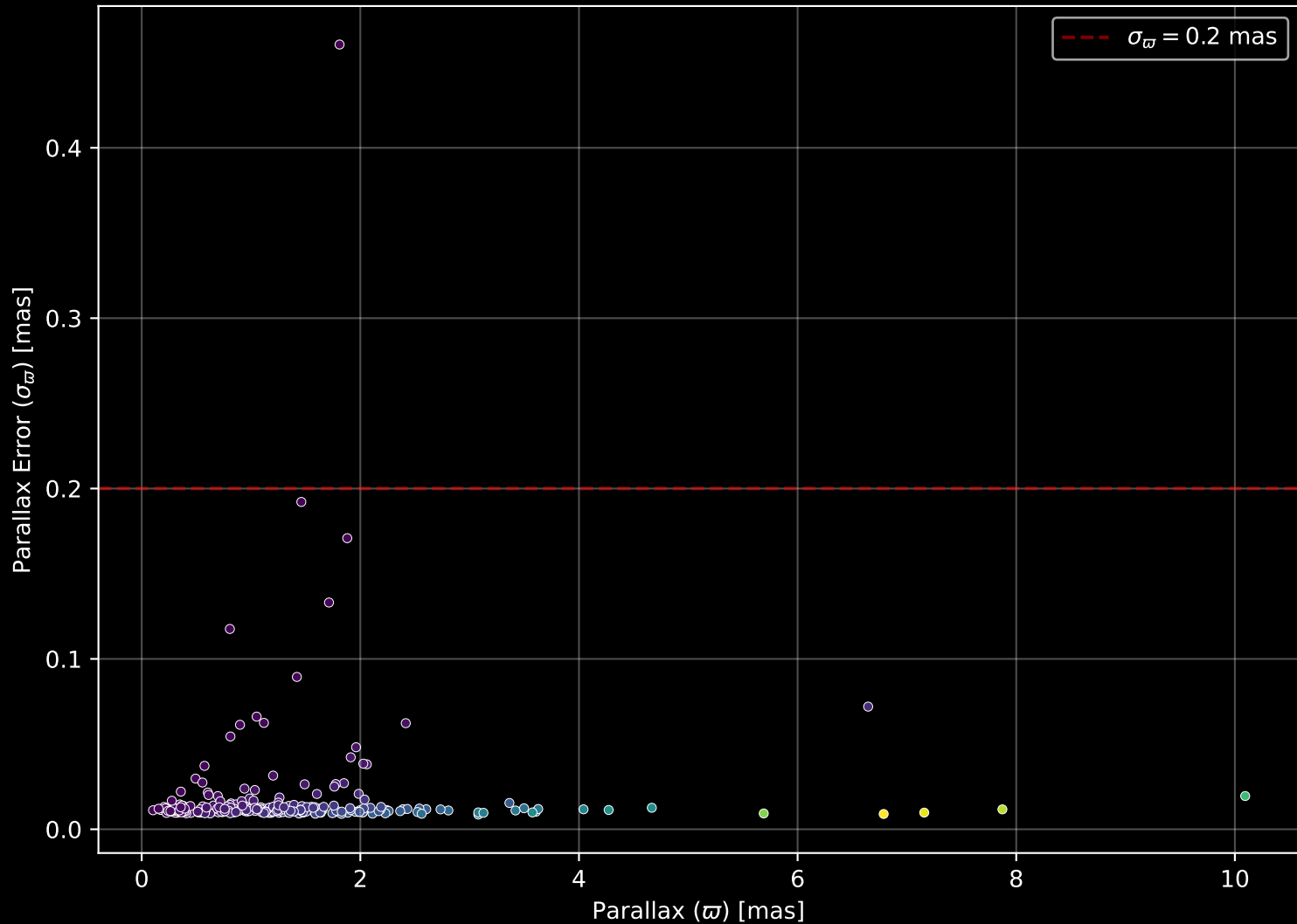
GALAH DR4 Field: [2848] Parallax Quality (n= 263)
