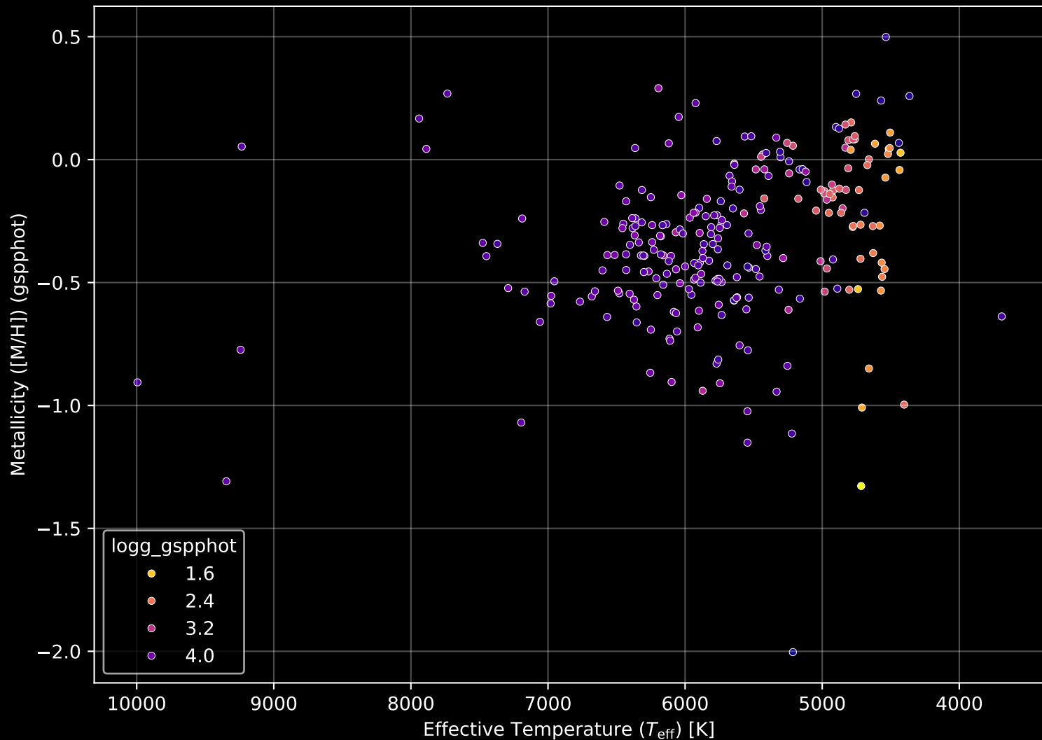
GALAH DR4 Field: [2848] Stellar Population Parameters (n= 263)
